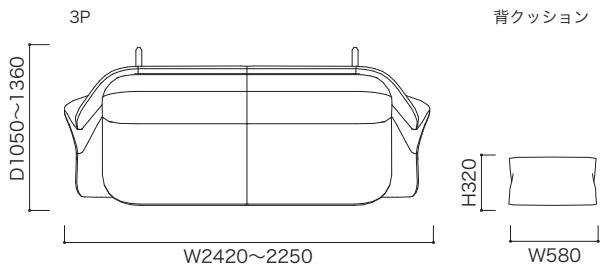
●平面図 1/50 (単位:mm)
